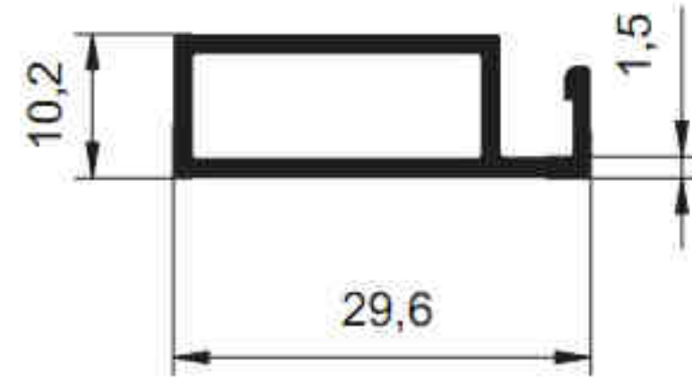
2862 - 0.284 kg/m
