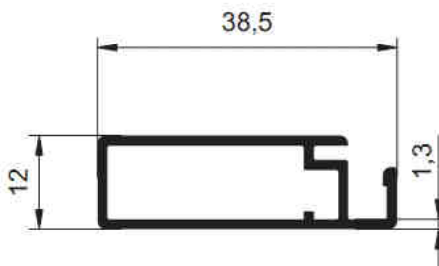
2860 - 0.359 kg/m
