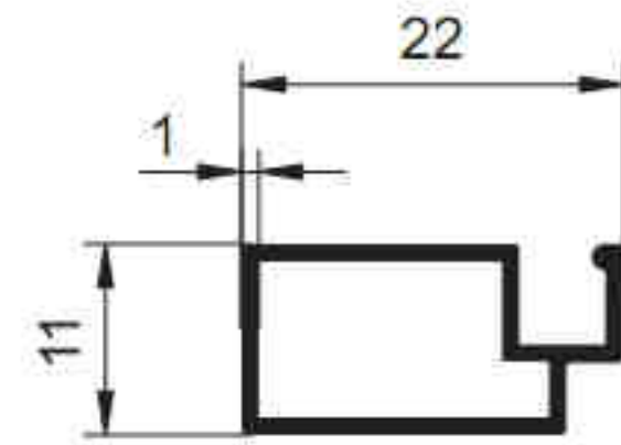
1483 - 0.178 kg/m
