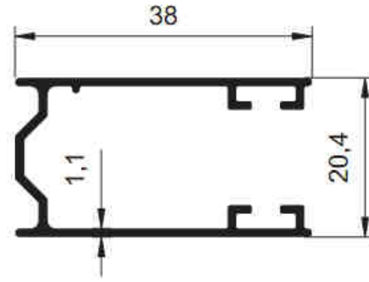
4662 - 0.354 kg/m
