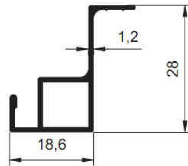
3741 - 0.270 kg/m
