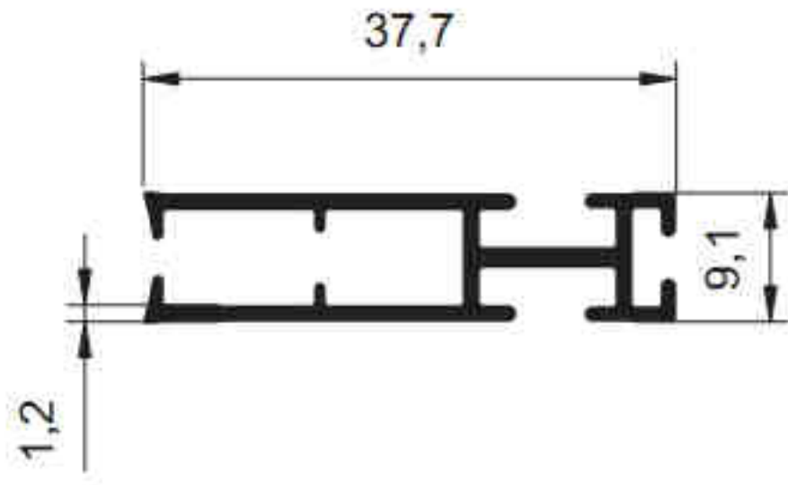
4661 - 0.320 kg/m
