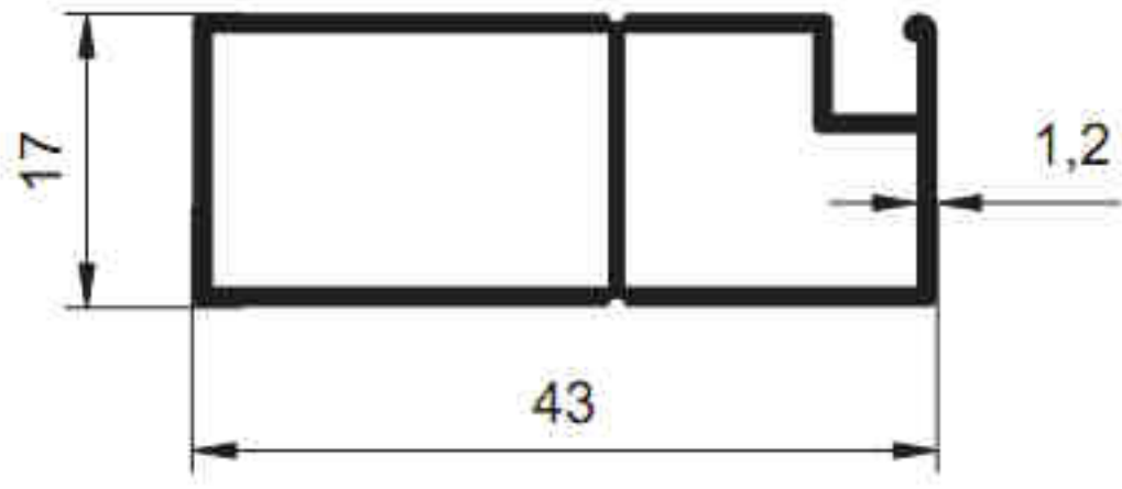
1662 - 0.430 kg/m
