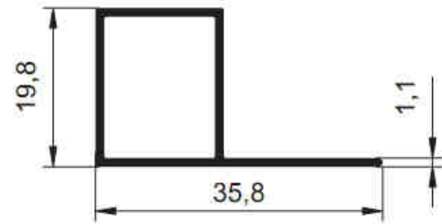
4659 - 0.257 kg/m
