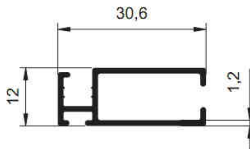
2845 - 0.267 kg/m
