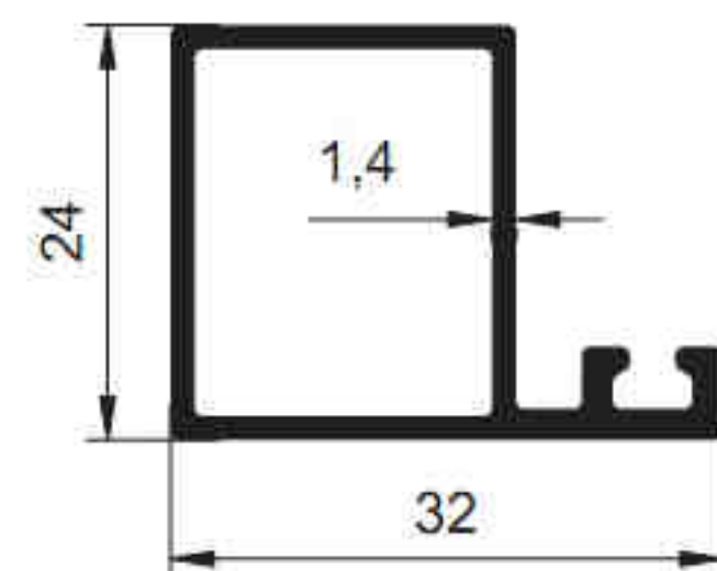
2764 - 0.521 kg/m
