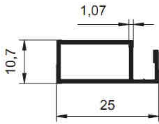
2742 - 0.203 kg/m
