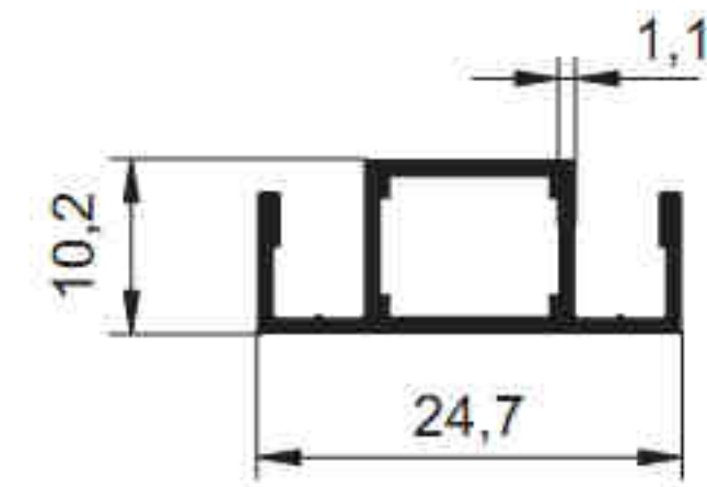
2745 - 0.203 kg/m
