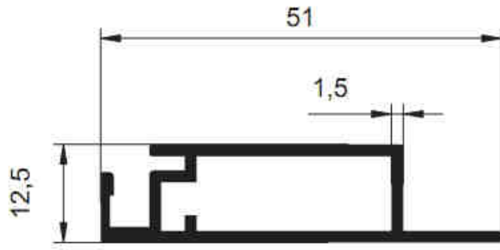
3742 - 0.475 kg/m
