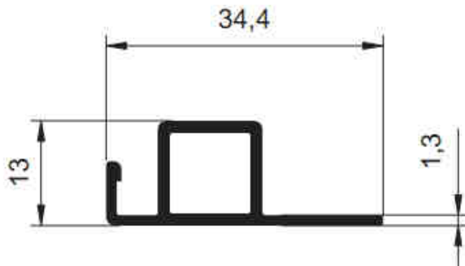
2861 - 0.287 kg/m
