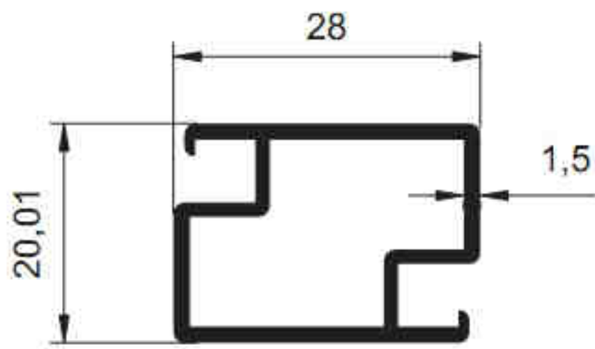
1386 - 0.404 kg/m
