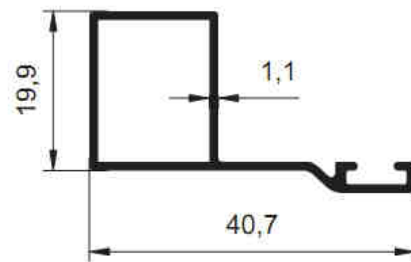
3332 - 0.305 kg/m
