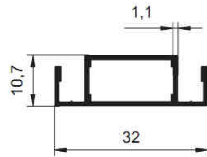
2744 - 0.257 kg/m
