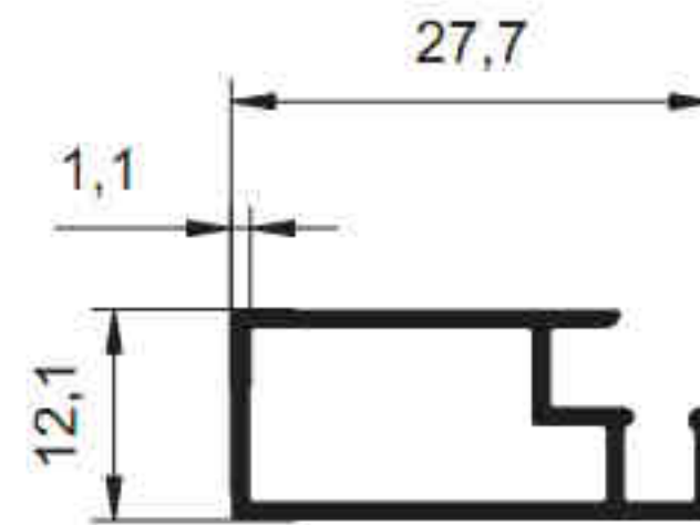
4660 - 0.238 kg/m
