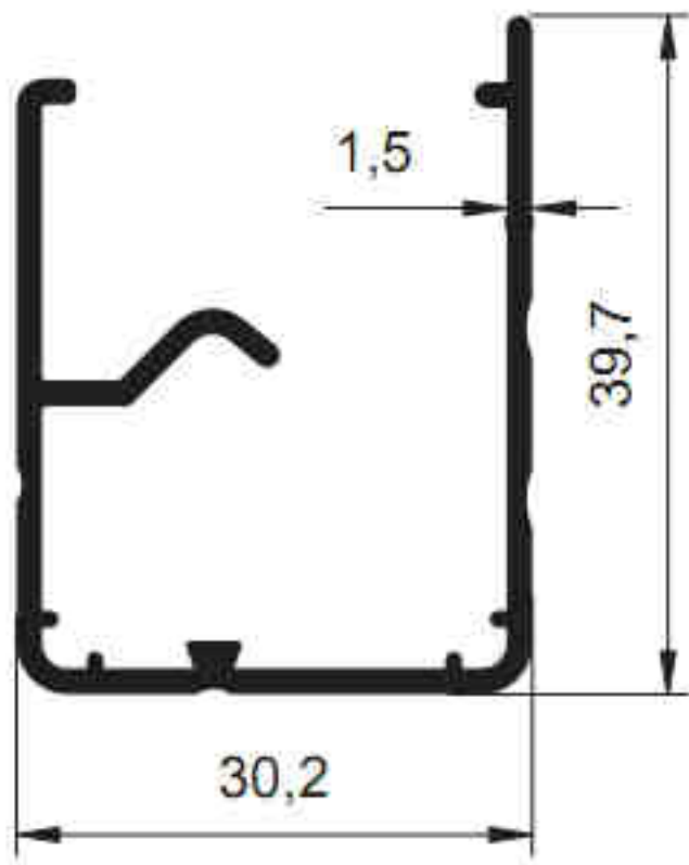
3334 - 0.502 kg/m
