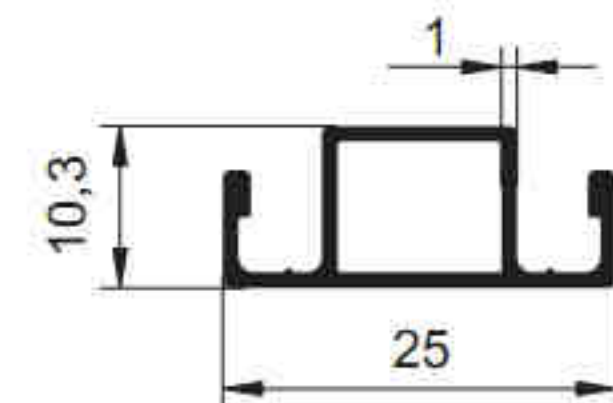
2771 - 0.196 kg/m
