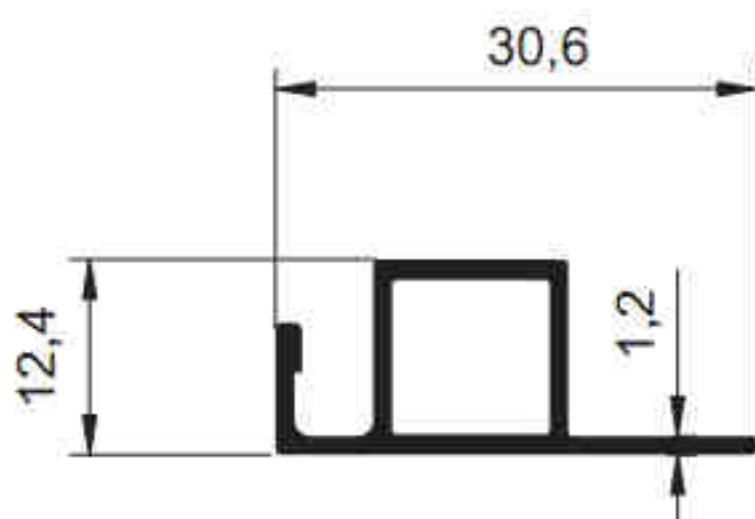
3765 - 0.238 kg/m
