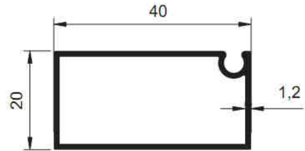
1385 - 0.391 kg/m
