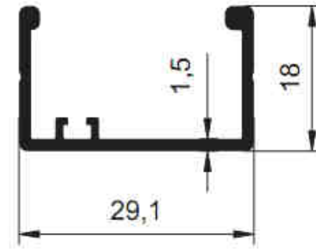
3335 - 0.290 kg/m
