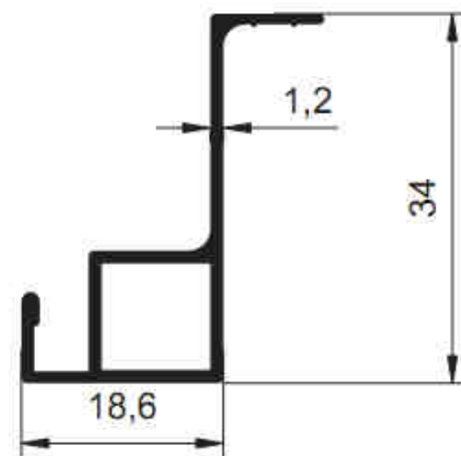
3740 - 0.289 kg/m
