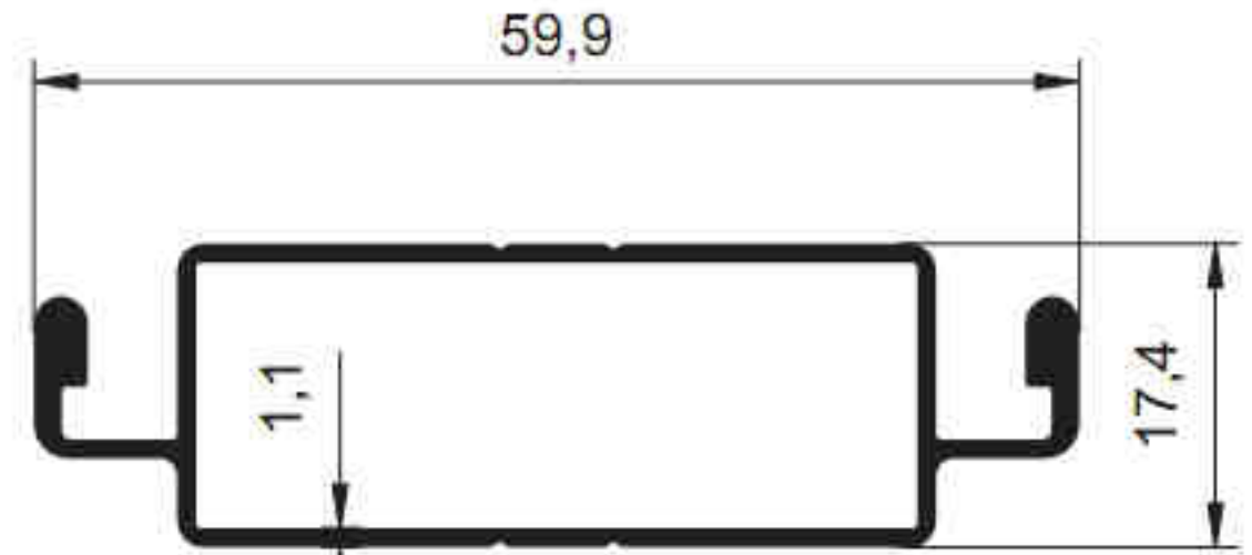
4664 - 0.494 kg/m
