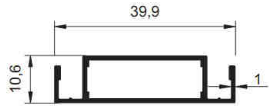
3506 - 0.304 kg/m
