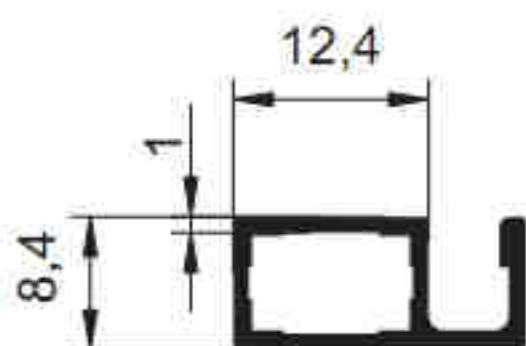
3503 - 0.158 kg/m
