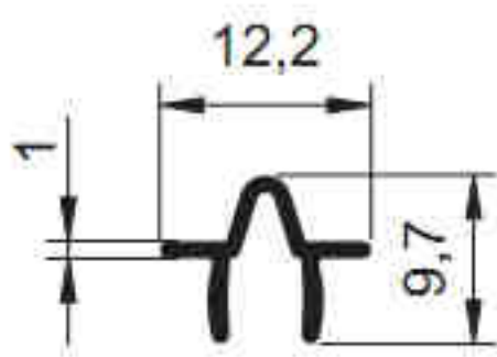
2852 - 0.076 kg/m
