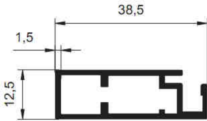
3739 - 0.443 kg/m
