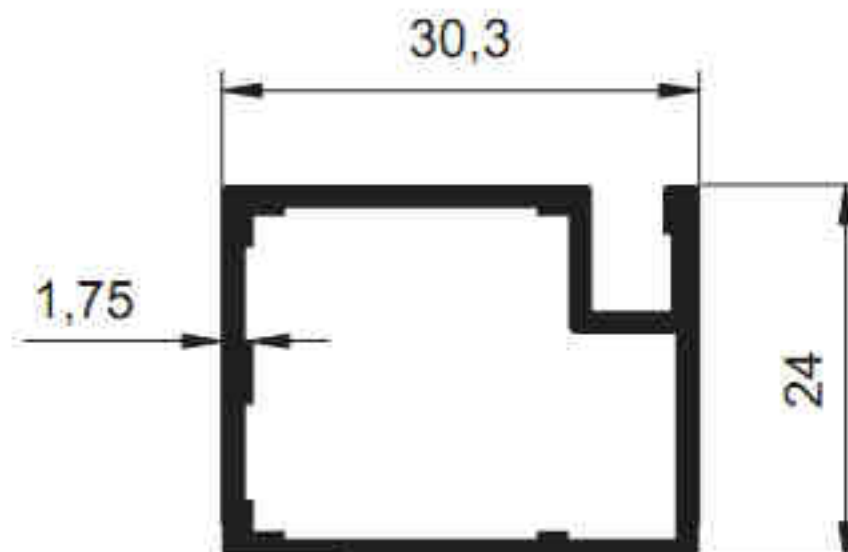
3745 - 0.481 kg/m
