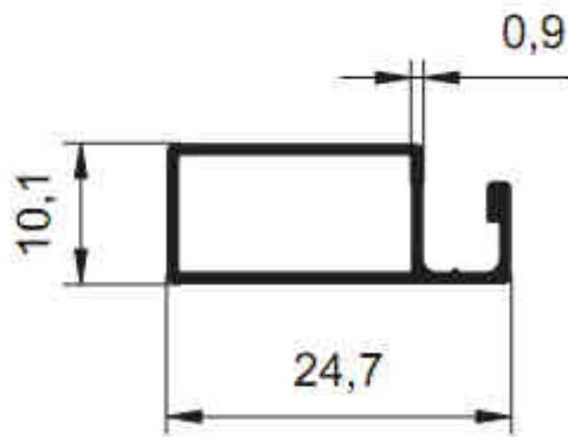
2723 - 0.169 kg/m
