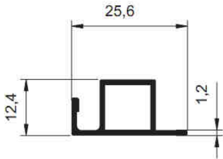
3743 - 0.221 kg/m
