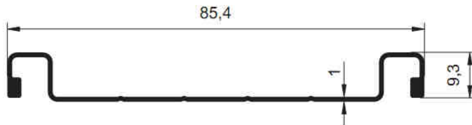
3336 - 0.356 kg/m
