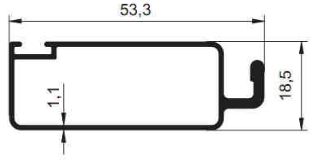
3333 - 0.476 kg/m
