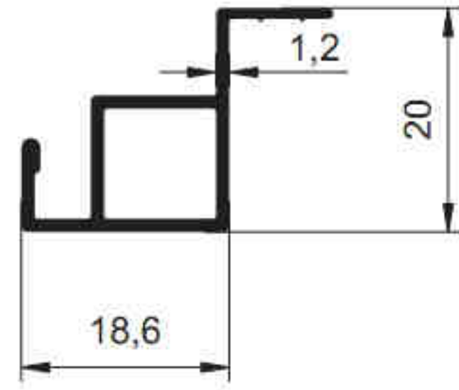
4119 - 0.240 kg/m
