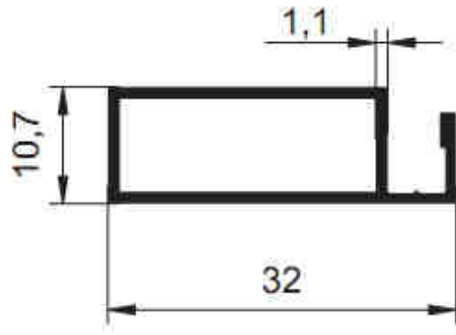
2743 - 0.245 kg/m
