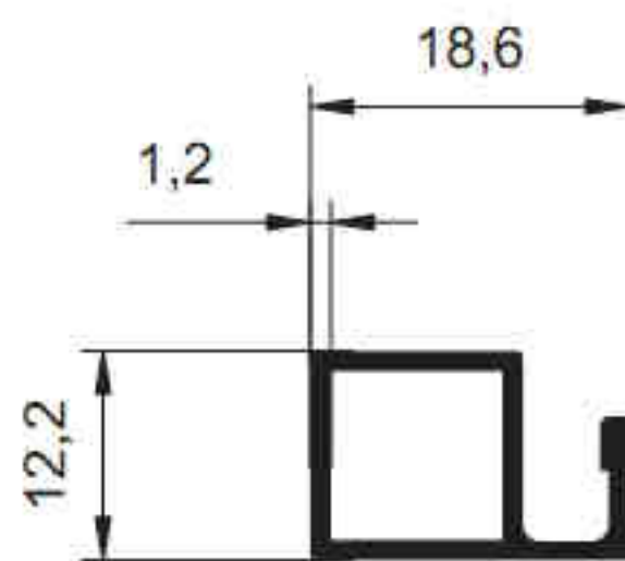
3744 - 0.191 kg/m
